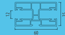
PG 02 Führung für Rollläden mit Teilung.
