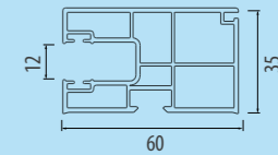
PG 08 Standardführung des Systems CleverBox.
