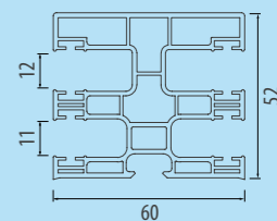
PG 09 Führung für Rollläden mit integriertem Moskitonetz.
