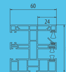
PVC PPDM 60/12 Führung für Rollläden Opoterm mit integriertem Moskitonetz. Verwendete Schrauben – RD2.
