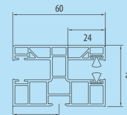
PVC PPD 60/12 Standardführung des Systems Opoterm. Verwendete Schrauben – RD2.
