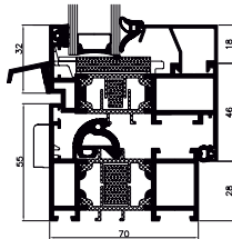
MB-70 HI Fenster Schnitt
