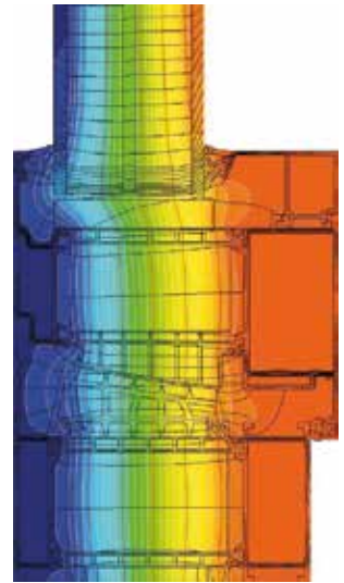
Isothermenverlauf im Fenster MB-104 Passive Aero
