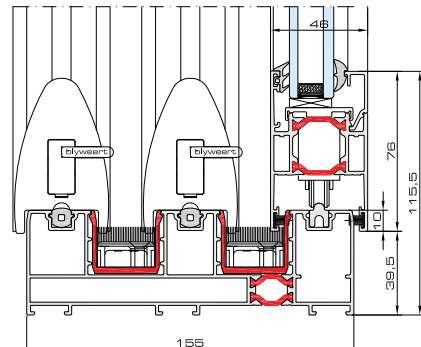
Notus mit drei Gleitschienen
