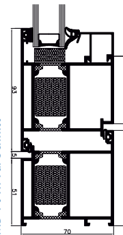
MB-70 HI Tür Schnitt
