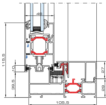
Notus mit einer Gleitschiene
