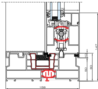
Kolos HI mit zwei Schienen vertikaler Querschnitt
