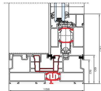
KOLOS HI mit zwei Schienen horizontaler Querschnitt
