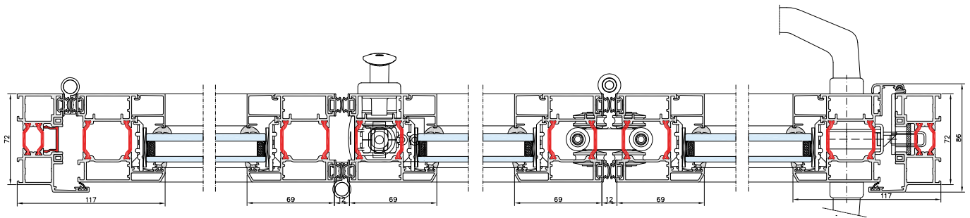
Querschnitt
