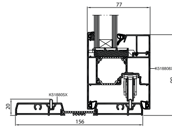
MB-77HS ST Flachschwelle Variante
